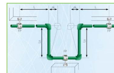
Hình 2. Vòng giãn nở Figure 1. Expansion ring
