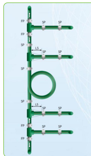
Ví dụ về bù giãn nở uốn tròn (Examples of circle bend compensation)
